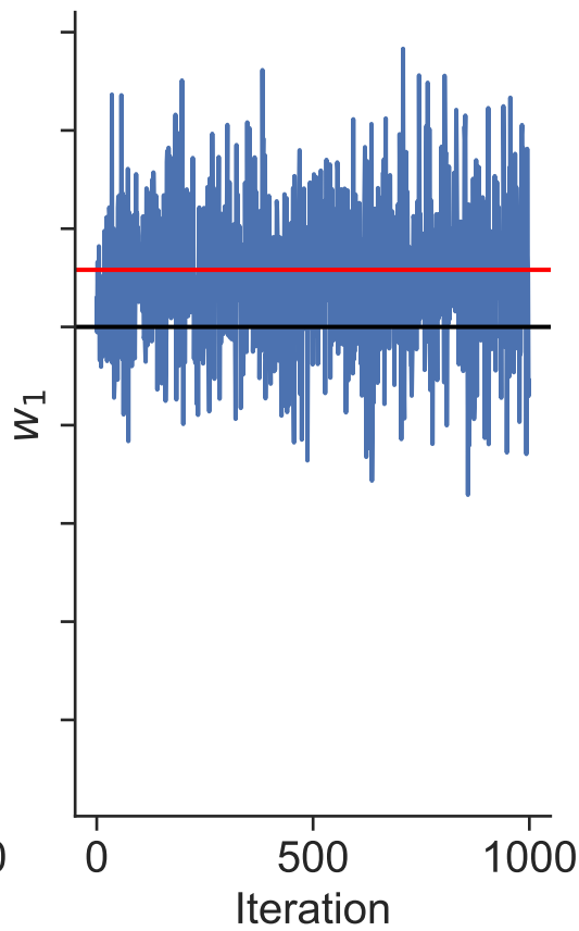
Posterior distributions Dataset 24
