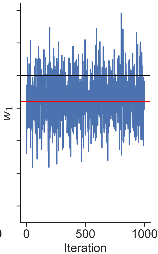
Posterior distributions Dataset 25
