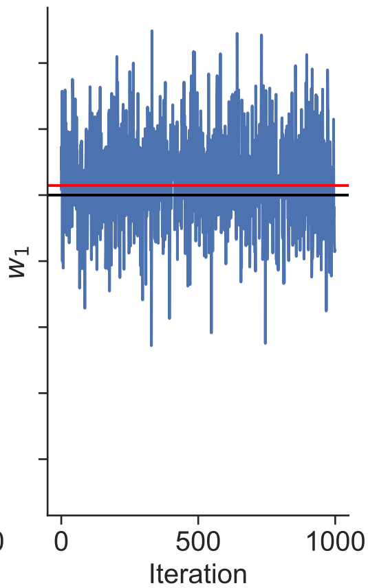
Posterior distributions Dataset 35
