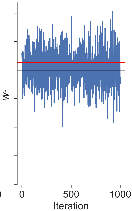
Posterior distributions Dataset 38
