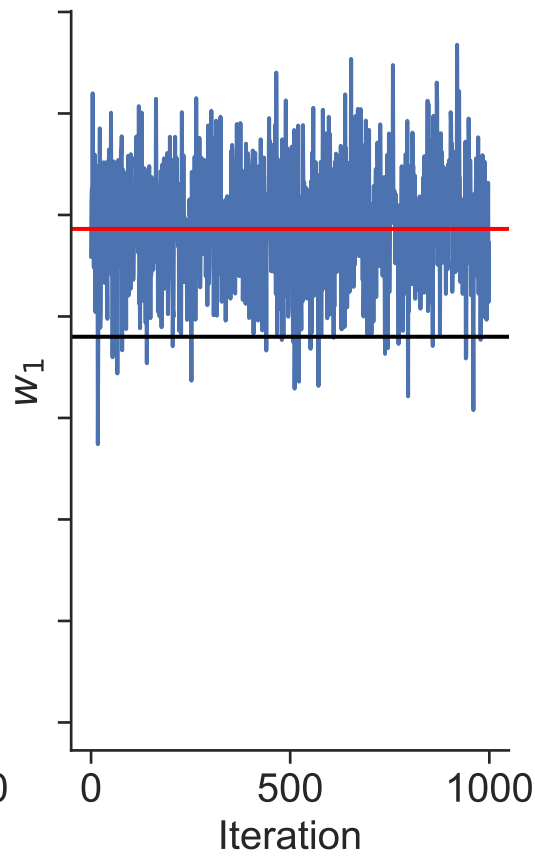
Posterior distributions Dataset 23
